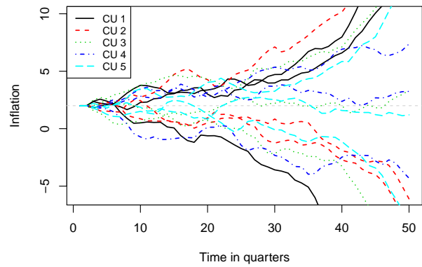
(d) Inflation, \Phi_\pi = 6 and \Phi_y = 2
